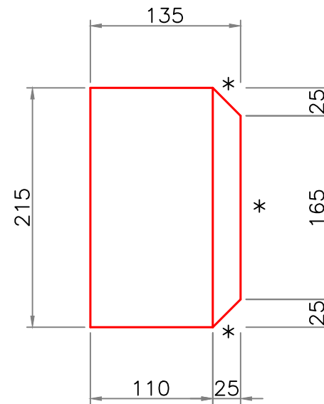
End Elevation
