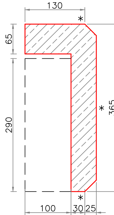
Section A-A
