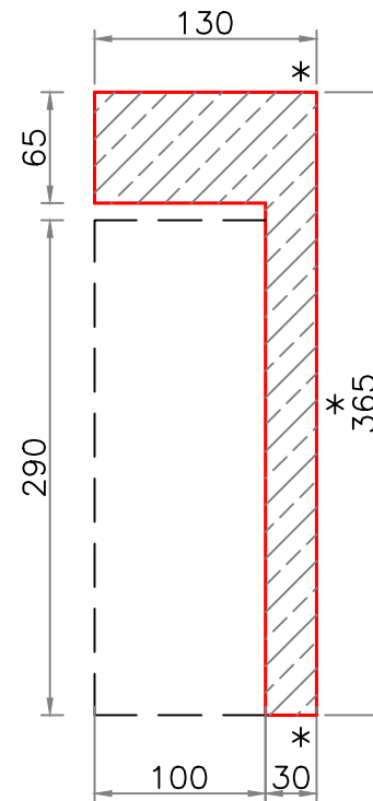
Section A-A
