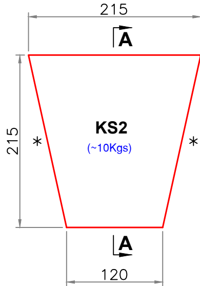
KS2 - Elevation
